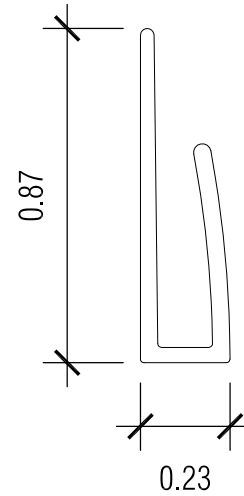
1 SIDE VIEW scale: 2:1
