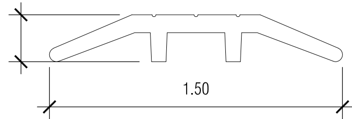
1 SIDE VIEW scale: 2:1
