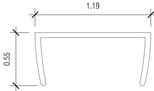
1 SIDE VIEW scale: 2:1
